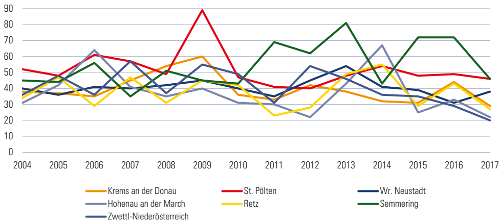
Tagesmaximum der Niederschlagshöhe pro Jahr (in mm) 2004–2017
