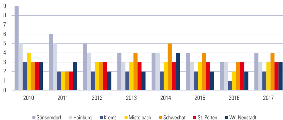
Schwefeldioxid – Jahresmittelwert ( \mu\text{g}/\text{m}^3 ) 2010–2017
