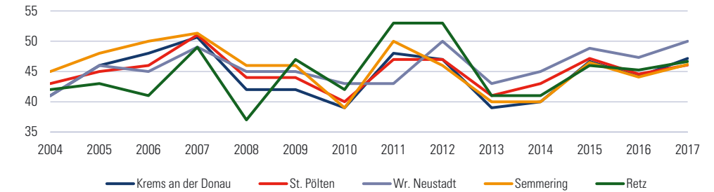
Sonnenschein in % der örtlich möglichen Dauer 2004–2017
