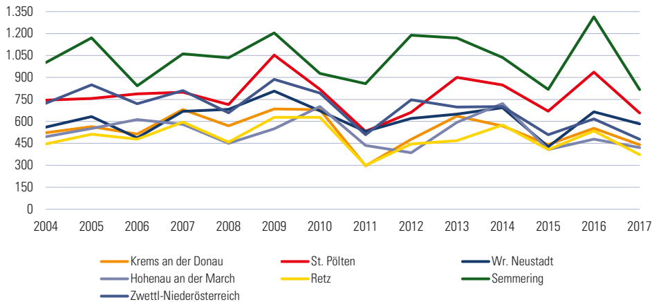
Jahresniederschlag (in mm) 2004–2017
