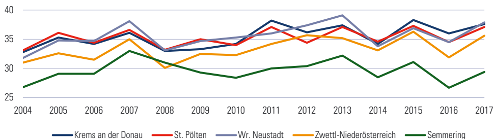
Höchste Lufttemperatur (in °C) 2004–2017
